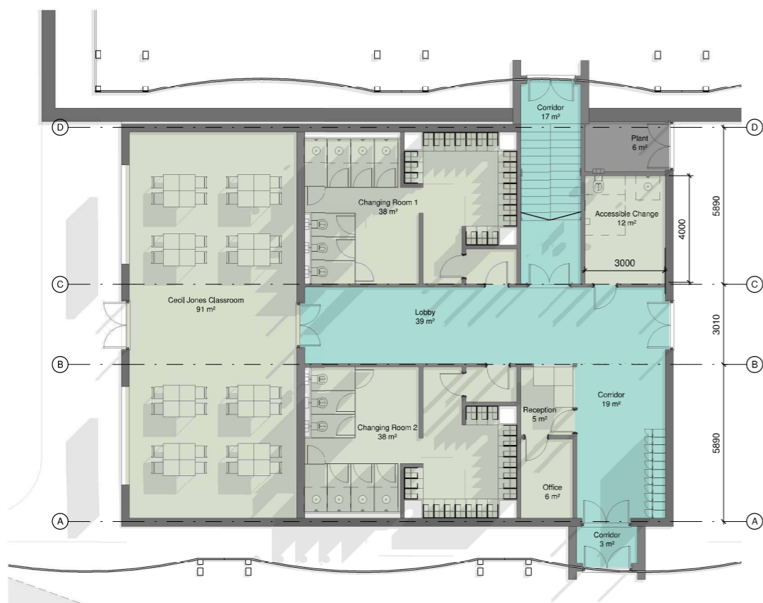
1 LOM 1 : 100
